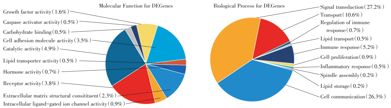
图2 差异表达基因 GO 分析结果
