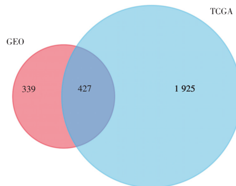
图1 TCGA数据库与GEO数据库中ccRCC差异表达基因韦恩图
