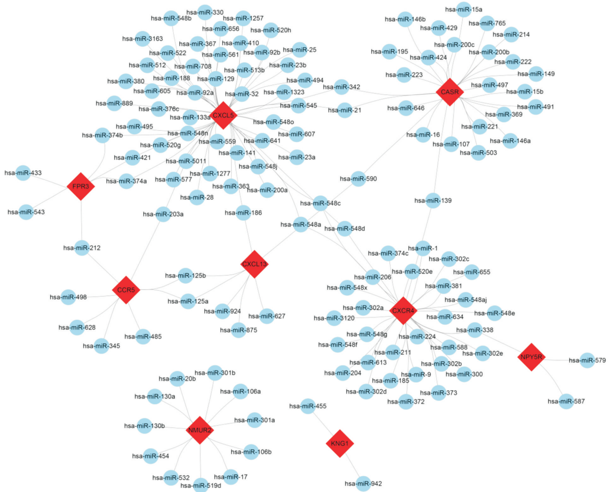
图4 核心基因及其对应 miRNA
