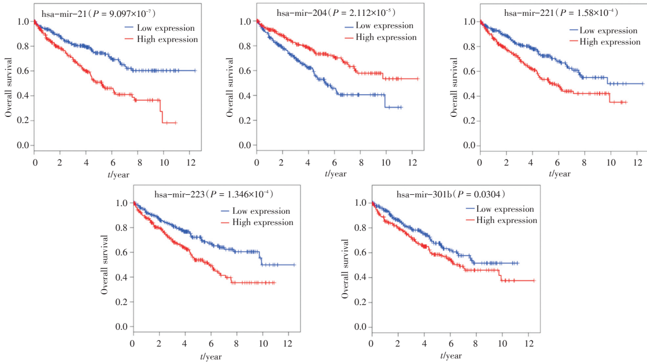
图5 miRNA 生存分析结果
